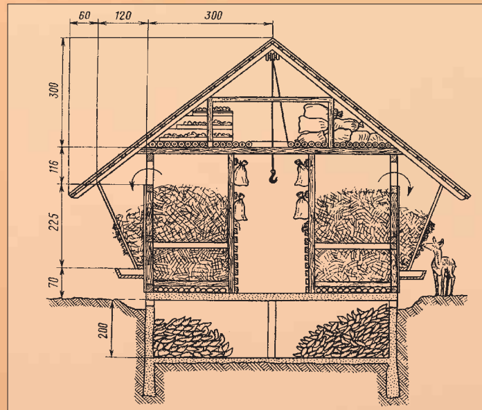
Kombinacija spremišta i hranilišta za izlaganje (spremanje) raznih vrsta hrane. Izvor: Kulich, 1975.
